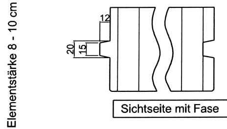
Profil 06: Nut und Feder
