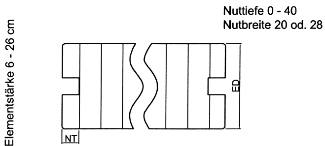
Profil 02: Nut und Falz
