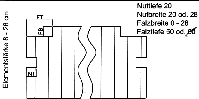
Profil 02: Nut und Falz
