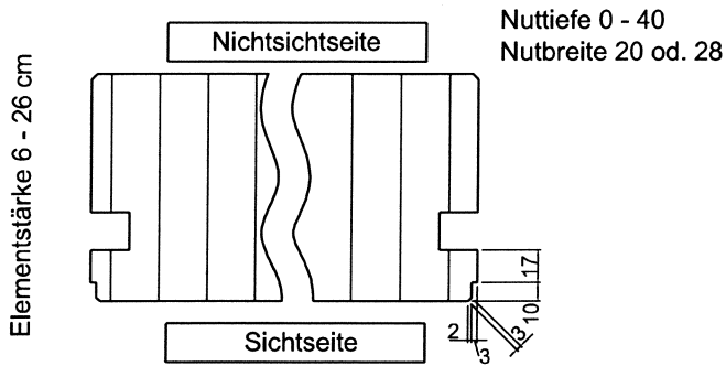
Profil 01: Nut mit Schattenfuge
