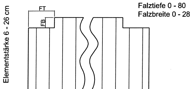
Profil 05: Falz
