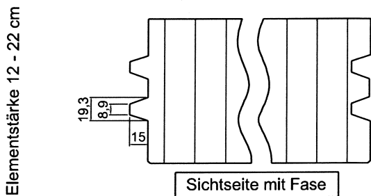
Profil 08: Doppelnut und Feder
