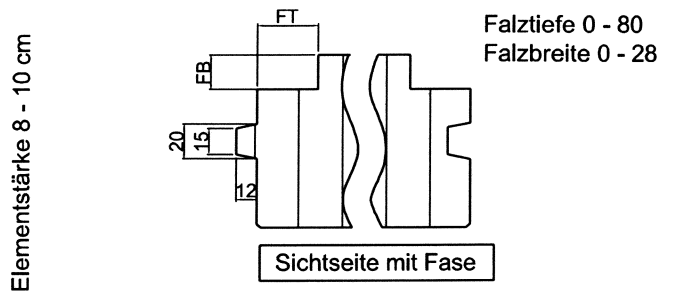
Profil 06: Nut und Feder
