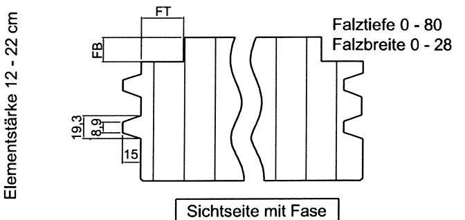
Profil 09: Doppelnut und Feder mit Falz
